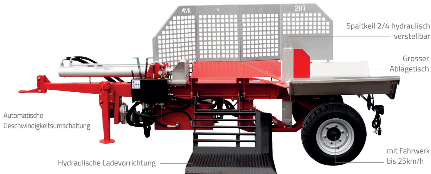
HPF28 ESS auf Fahrwerk
